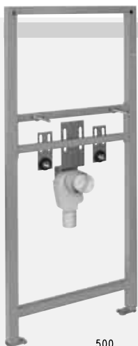
Waschtisch-Element
