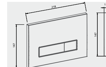
TREND glanz verchromt / schwarz Art.-Nr. 167-32003618-00
